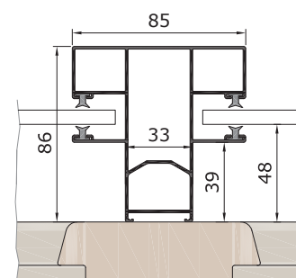
Führungsschiene KD85K / * GD85K
