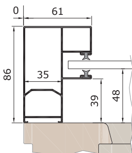
Führungsschiene KD61K / * GD61K
