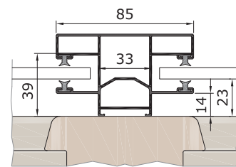
Führungsschiene KE85K / * GE85K
